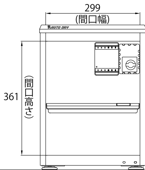
正面図(扉開放時)
