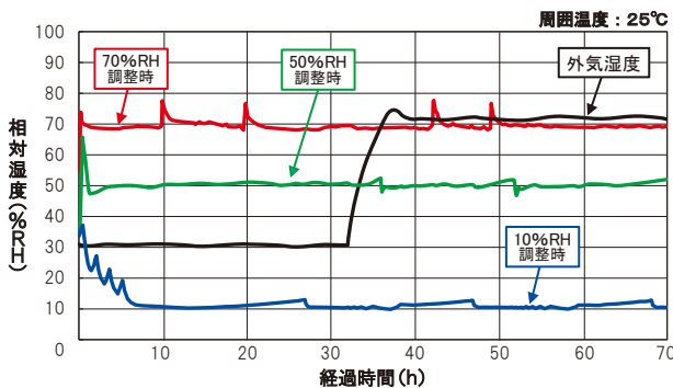
FD-1206F1 設定湿度別 性能試験データ
