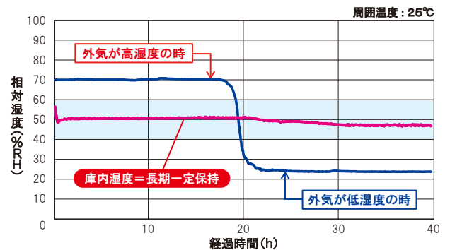
FD-502F1 連続運転試験データ
